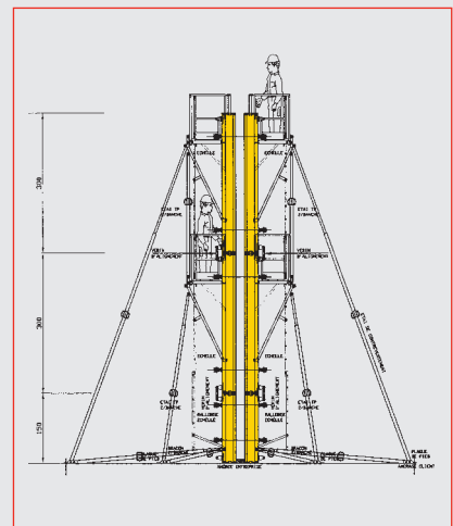
Exemple de banches H : 7,50 m.
